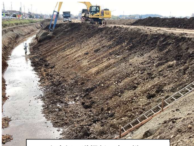
右岸側河道掘削工事の様子
