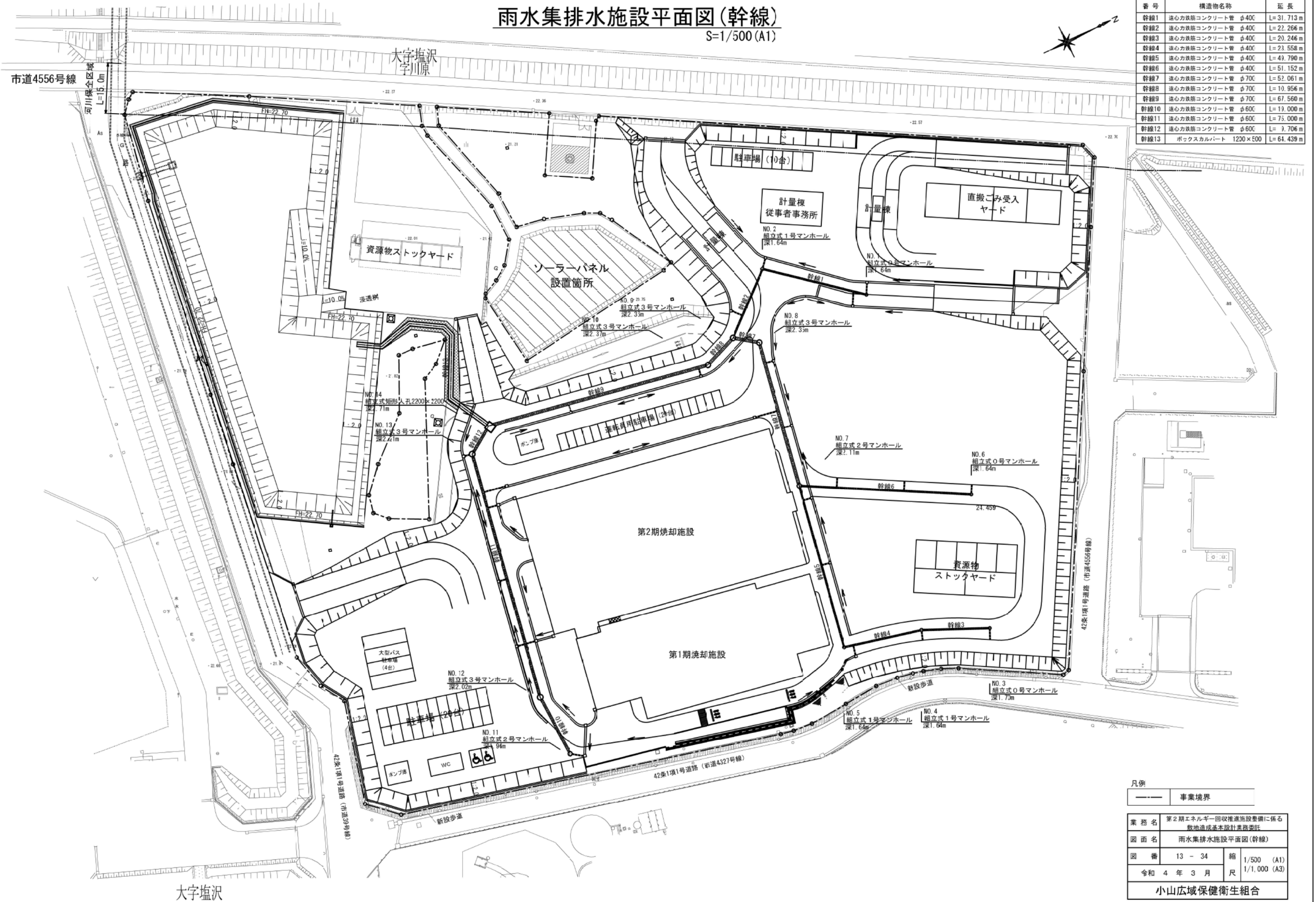
図 2-2-5 雨水集排水施設平面図(幹線)
