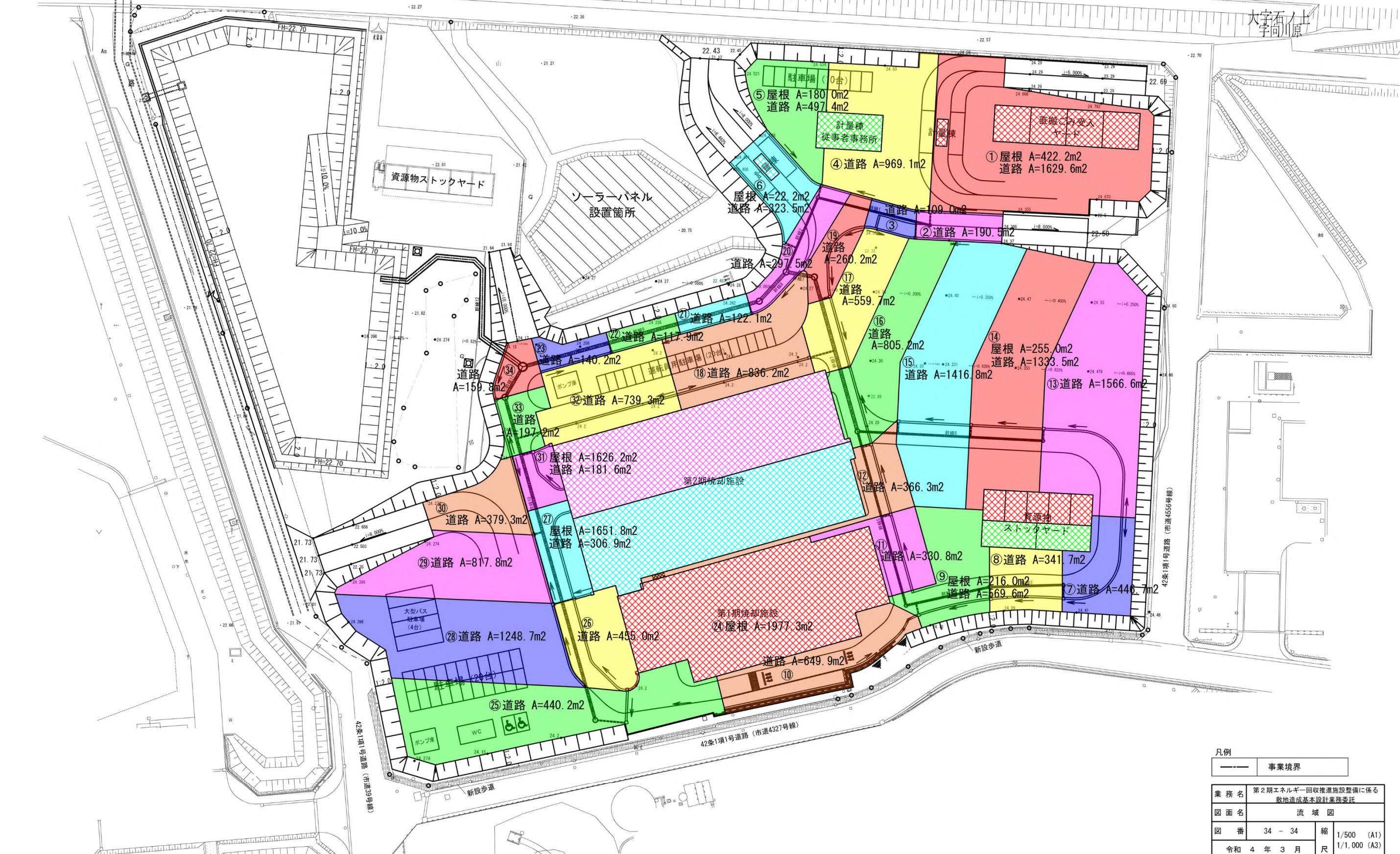
図 2-2-3 流域図
