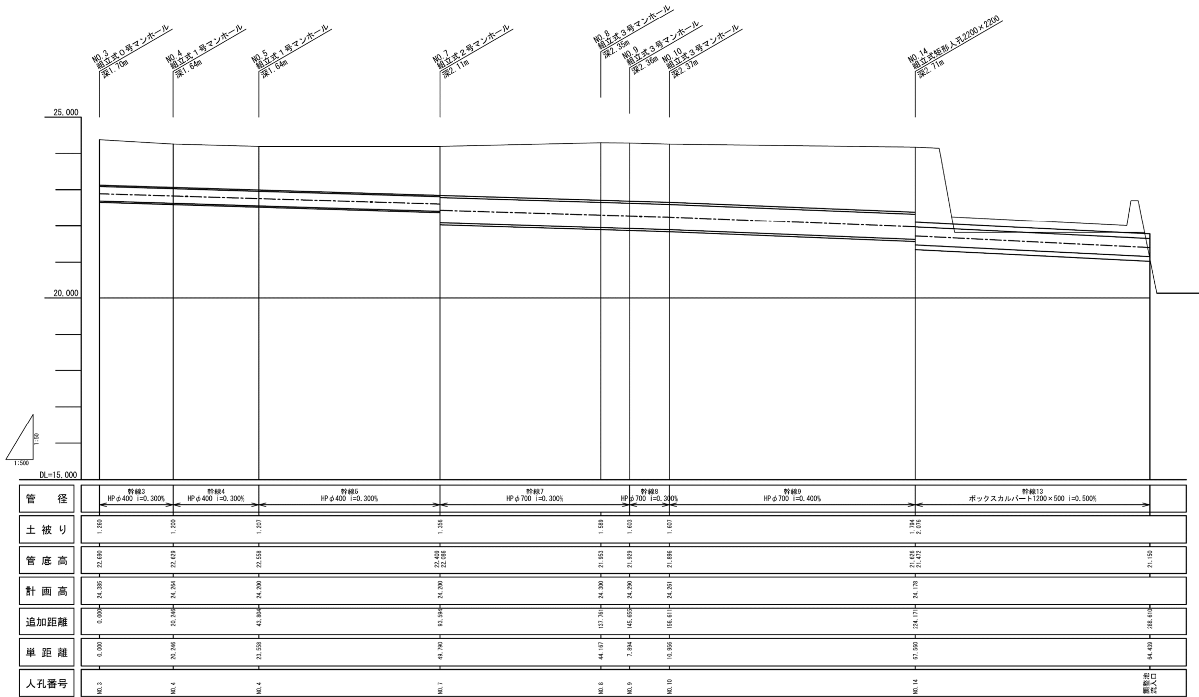
図 2-2-6 雨水幹線縦断面図（１）
