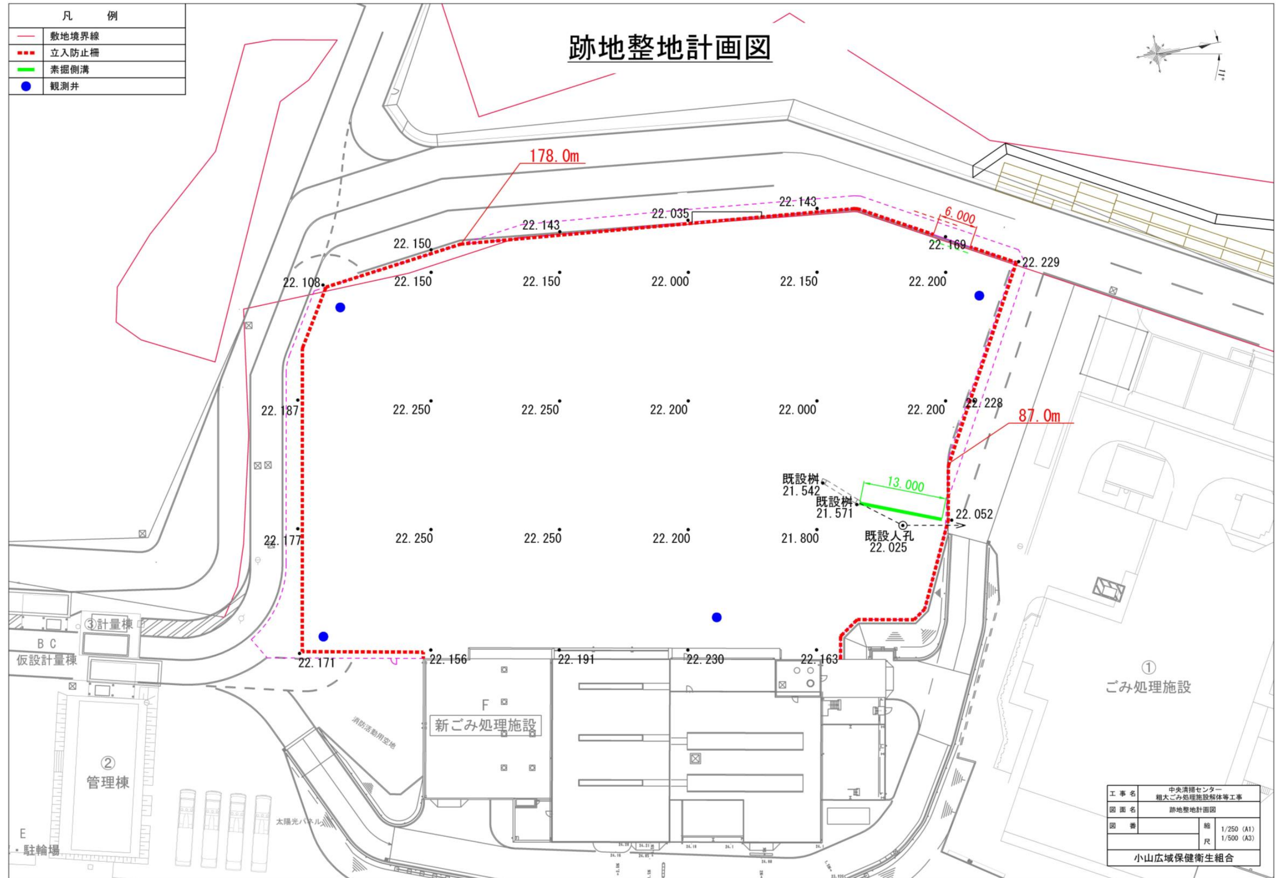
図5-1 跡地整地計画図（整地工、立入防止柵工、素掘側溝工）
