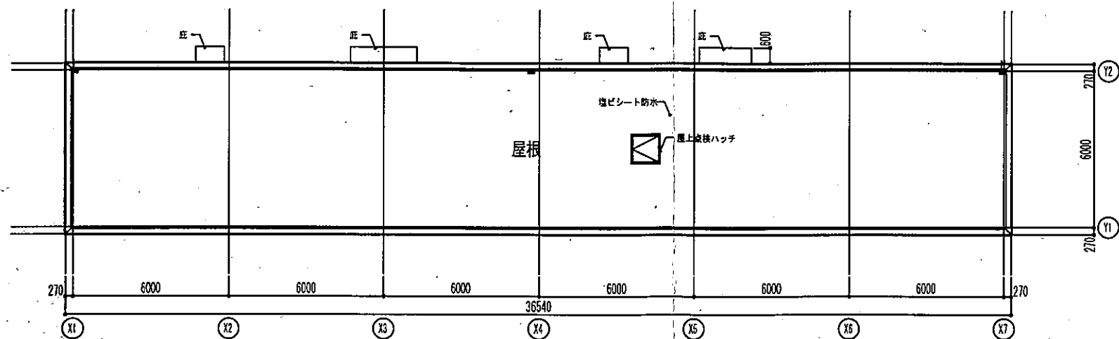
RF 平面図
