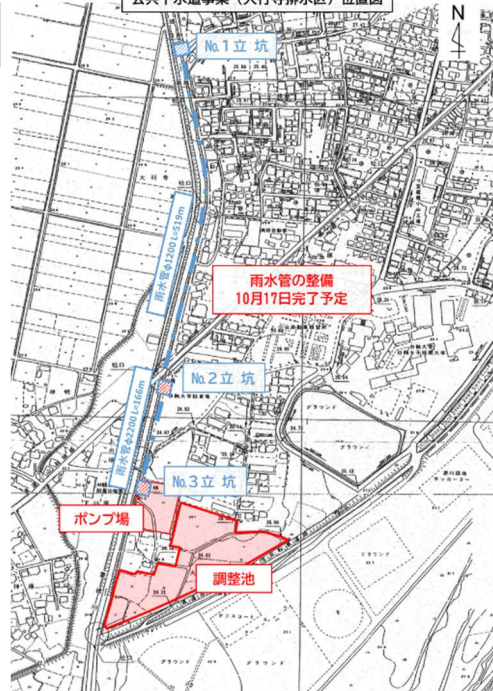
公共下水道事業（大行寺排水区）位置図
