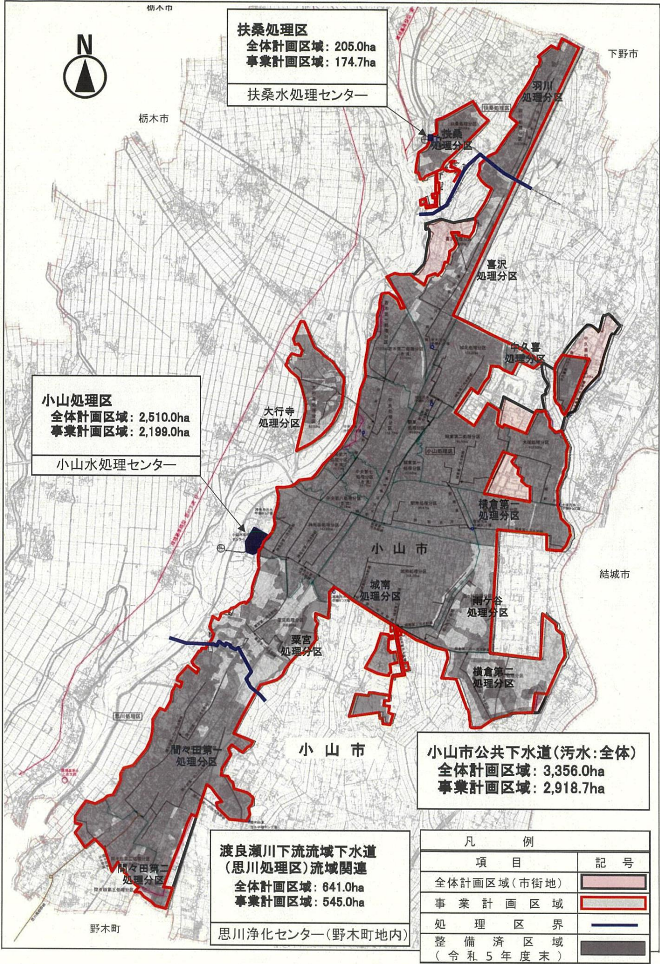
(3) 公共下水道（污水）整備状況図
