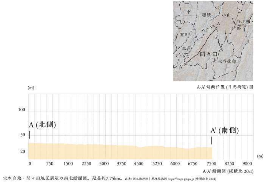
宝木台地・間々田地区周辺の南北断面図。延長約7.75km。出典：国土地理院 | 地理院地図 https://maps.gsi.go.jp/ (廣瀬改変 2024)
