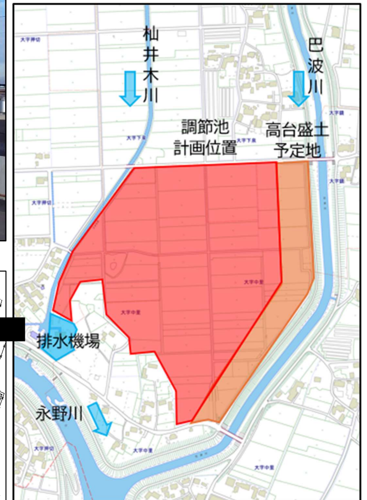
杣井木川の調節池の整備計画図(完成形)
